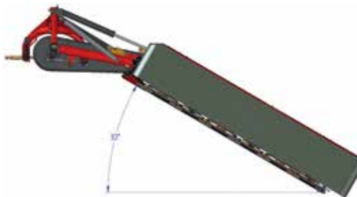
Enganche de tres puntos lateral: posibilitar cortes en terrenos con pendiente.
